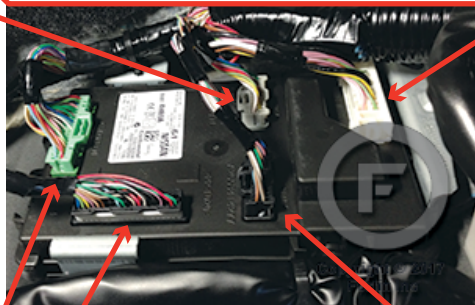
BCM located behind instrument cluster BCM Situé derrière l'odmètre
