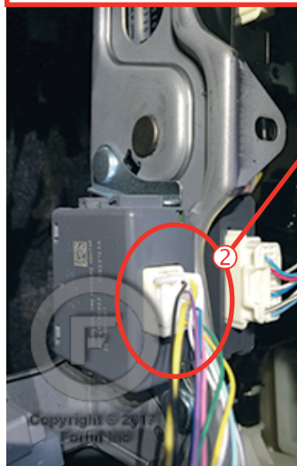
② TPMS module behind glove box. Module TPMS derrière la boîte à gant
