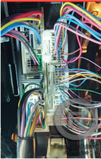
③ ECU left of the steering column ECU à gauche de la colonne de direction
