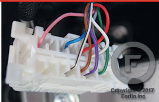
④ OBD-II connector Connecteur OBD-II
