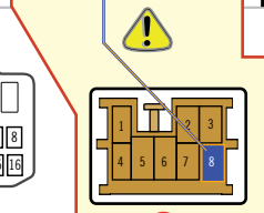
4 White connector At Push-to-Start button 8pin Back View Au dos du bouton Push-to-Start Connecteur Blanc - 8-pin Vue de dos.
