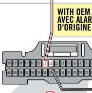
1 BCM Black 40-Pin Connector Back view BCM Connecteur Noir de 40-Pin Vue de dos
