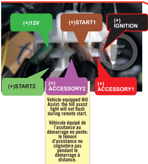
① Ignition harness Connecteur d'ignition
