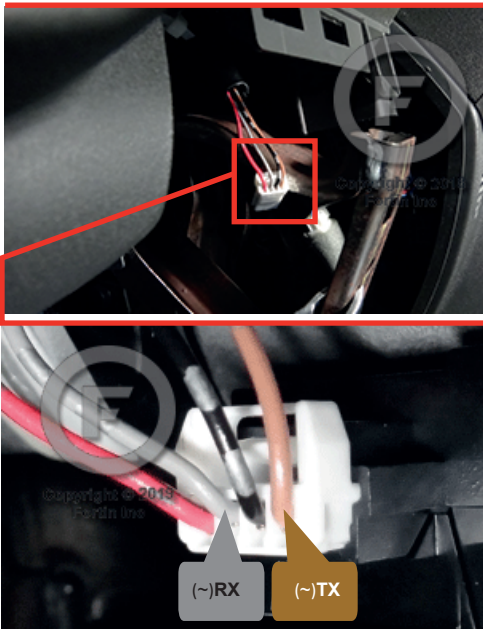
② Transponder connector Connecteur du transpondeur
