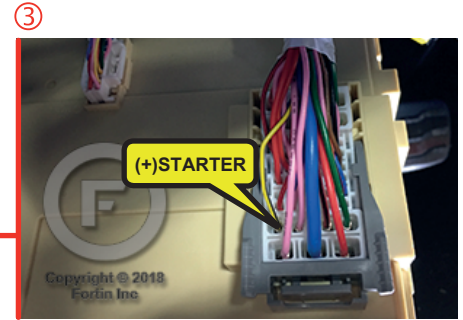
③ Rear of the Fusebox/Smart Junction Box Dos de la boîte à fusibles/Smart Junction
