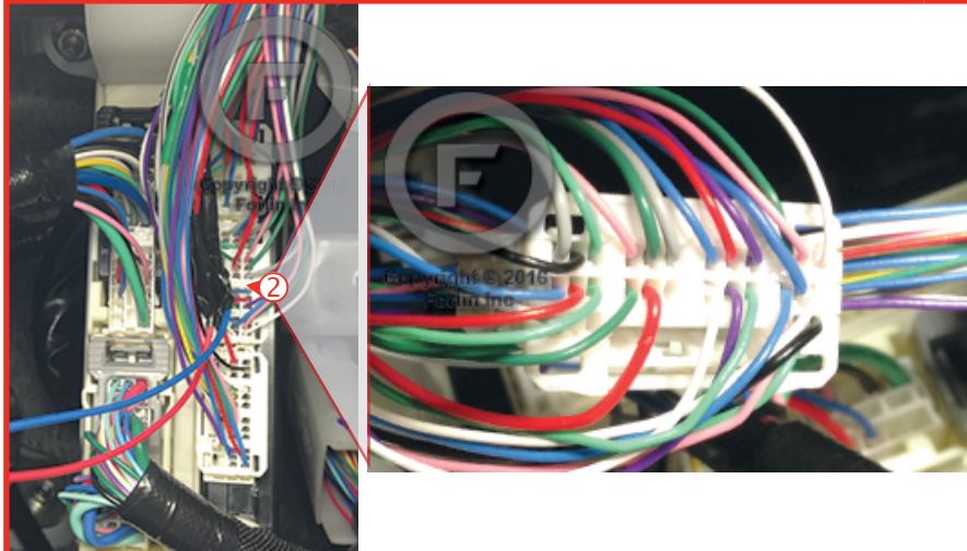
② MAIN BODY ECU LEFT SIDE OF THE DASH CÔTÉ GAUCHE DU TABLEAU DE BORD
