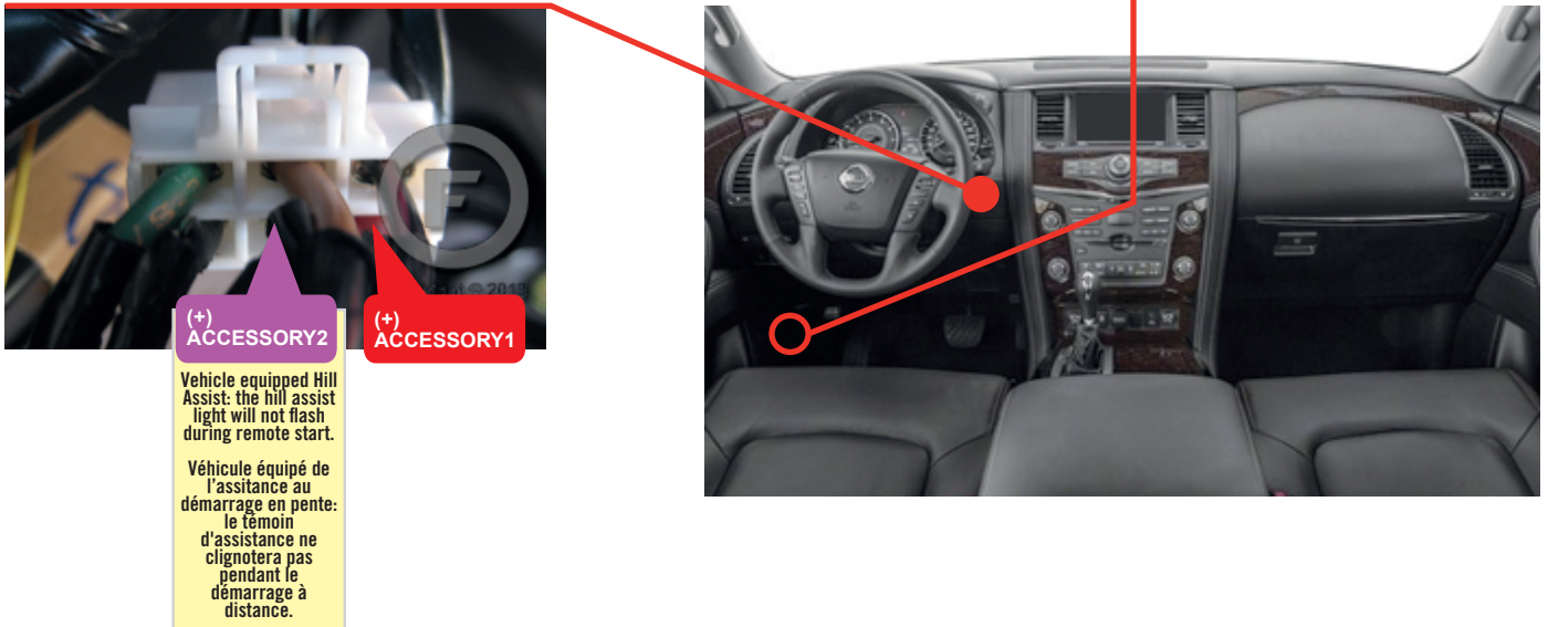
① Ignition harness Connecteur d'ignition
