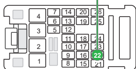
① Back view, 26-Pin White connector, at BCM. Vue de dos, connecteur Blanc 26-Pins, au BCM.
