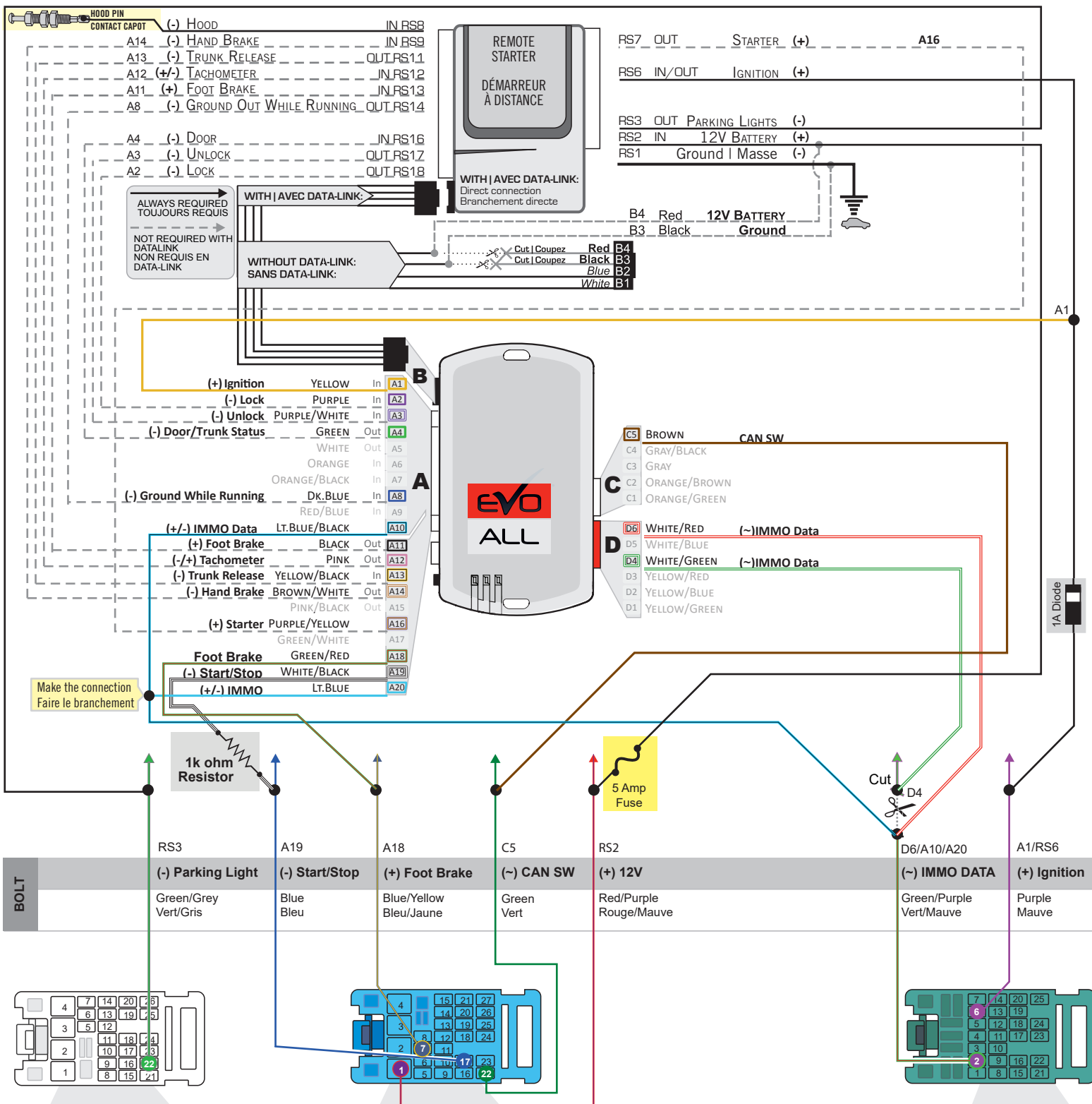
① Back view, 26-Pin White connector, at BCM. Vue de dos, connecteur Blanc 26-Pins, au BCM.
