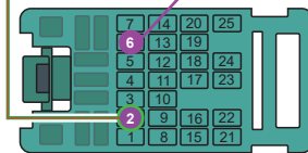
③ Back view, 25-Pin Green connector, at BCM. Vue de dos, connecteur Vert 25-Pins, au BCM.
