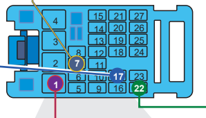
② Back view, 27-Pin Blue connector, at BCM. Vue de dos, connecteur Bleu 27-Pins, au BCM.
