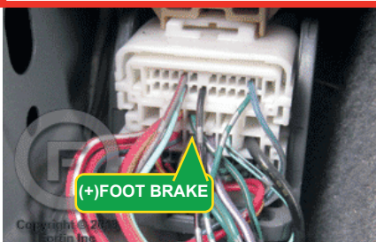
At Driver's kick panel Au Panneau latéral côté conducteur
