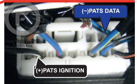
③ At Module at the right of the steering column Au Module à droite de la colonne de direction
