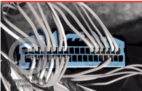
② BCM Blue 36-PINS connector. BCM Connecteur Bleu de 36-PINS.
