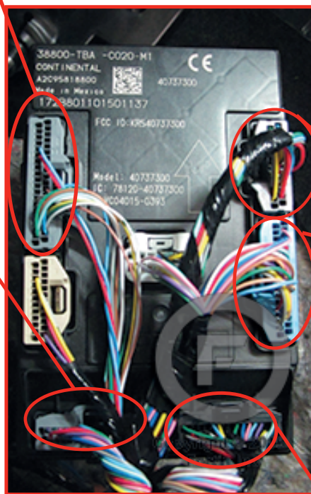
④ BCM Blue 36-PINS connector. BCM Connecteur Bleu de 36-PINS.
