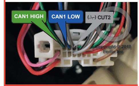
⑤A Back of the fuse box Au dos de la boîte à fusibles
