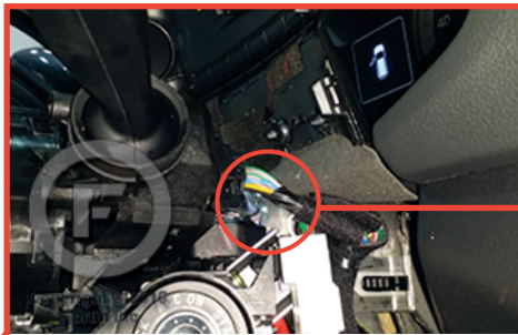
③ Steering column. À la colonne de direction.
