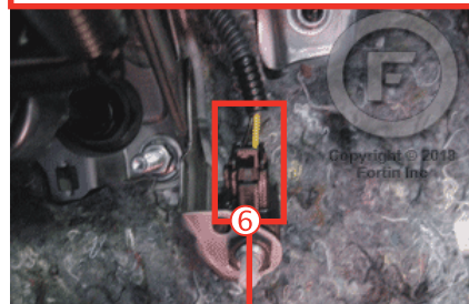
⑥ At Clutch switch Au Commutateur d'embrayage
