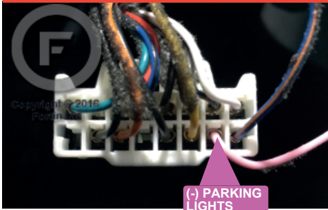
② Driver kick panel Panneau latéral côté conducteur
