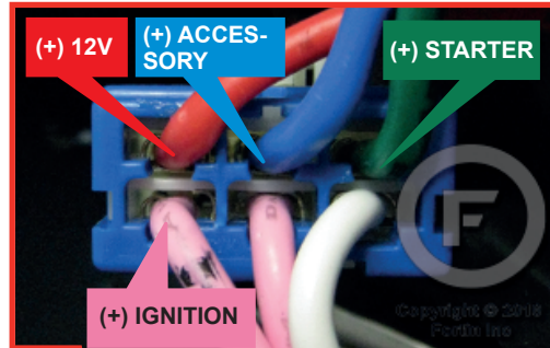
Ignition harness Harnais d'ignition
