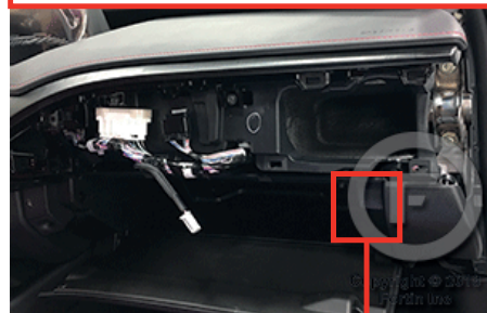
② ⑥ ECU, behind glove box ECU, derrière le coffre à gants
