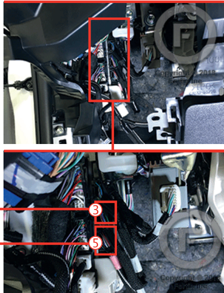
③ ⑤ ECU, driver's side ECU, côté conducteur
