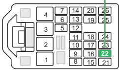
① Back view, 26-Pin White connector, at BCM. Vue de dos, connecteur Blanc 26-Pins, au BCM.
