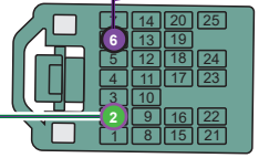
③ Back view, 25-Pin Green connector, at BCM. Vue de dos, connecteur Vert 25-Pins, au BCM.
