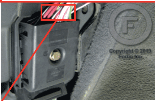
⑥ Harness from driver door Harnais de la portière côté conducteur
