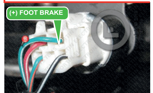
⑦ At Brake switch Au Commutateur de frein
