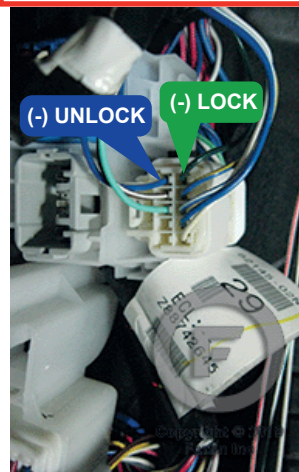
⑤ At Driver's kick panel Au Panneau latéral côté conducteur
