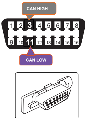
④ OBDII
