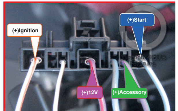
② Harnais d'ignition Ignition harness
