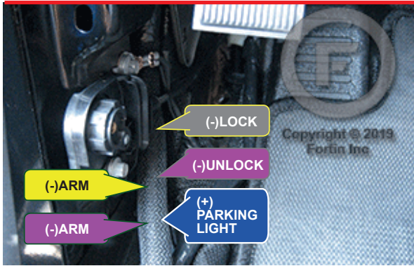
⑤ Driver kick pannel Panneau latérale côté conducteur
