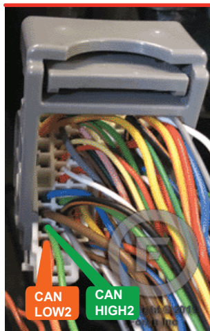
①B Driver's side kick panel Panneau latéral côté conducteur
