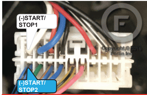
③ Start Stop Button Switch Commutateur du bouton démarrage
