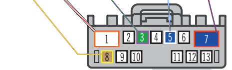
① At ignition barrel Black ignition connector (13-pins) Back view Au barillet d'ignition connecteur Noir d'ignition (13-pins) Vue de dos
