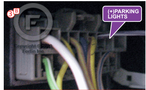
③ BCM Driver kick panel BCM Panneau latérale côté conducteur
