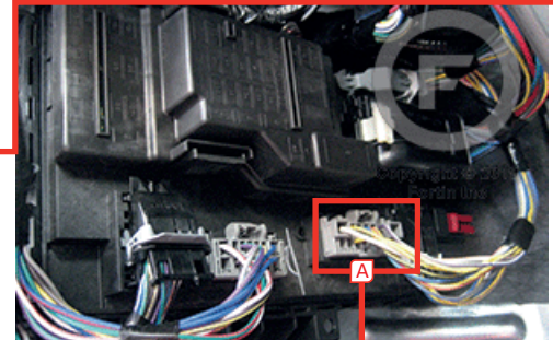
③ Smart Junction Box, Connecteur A Boîte de Jonction est situé dans le Panneau Latéral Conducteur
