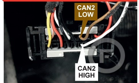
③ OBDII connector Connecteur OBDII
