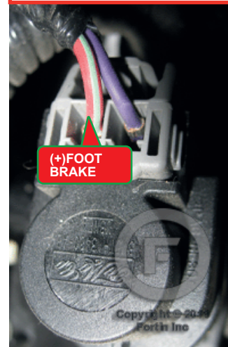
④ Brake switch Commutateur de frein
