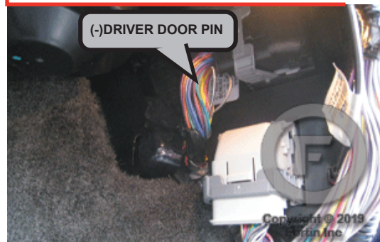
⑤ At passenger kick panel Au panneau latéral côté passager
