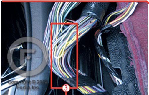
③ Driver running board harness Harnais au panneau courant du conducteur
