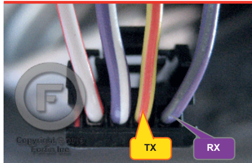
① transponder connector - Ignition barrel. Connecteur transpondeur - Barillet d'ignition.
