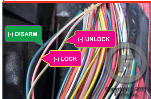
⑤ Harness from driver door Harnais de la portière côté conducteur
