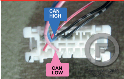
④ OBDII
