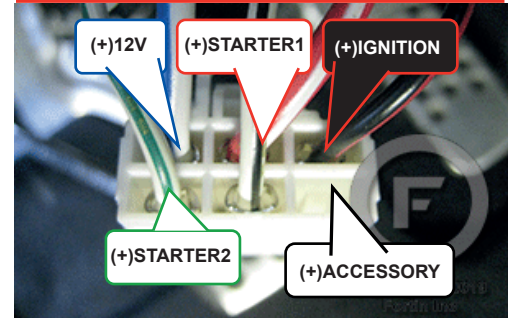
① Ignition harness Connecteur d'ignition
