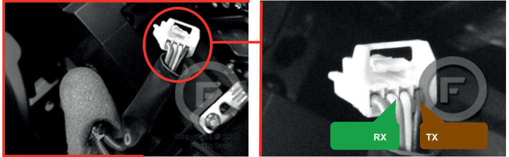
② Transponder connector Connecteur du transpondeur
