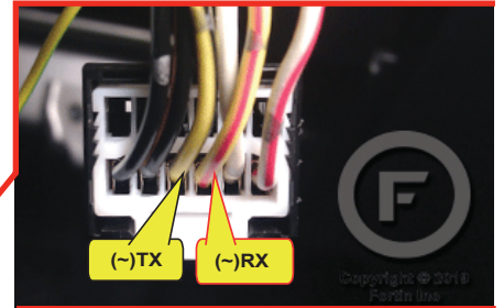
③ At Transponder Au Transpondeur
