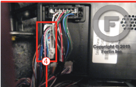
④ BCM connector Connecteur BCM
