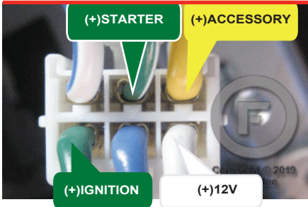
① Ignition connector Connecteur d'ignition
