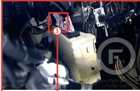
③ Behind Fusebox, driver side dash. Sous la boîte à fusibles, tableau de bord côté conducteur.
