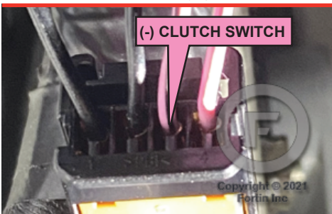
⑤ Clutch switch Commutateur d'embrayage
