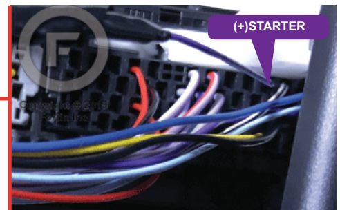
Steering Lock Connector Connecteur Steering Lock
