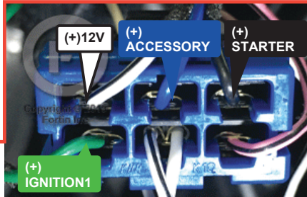
② Ignition Harness Harnais d'ignition
