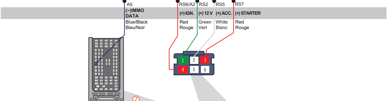
② Back view - Grey 82-pin connector - In the driver's side kick panel Vue de dos - Connecteur Gris de 82-pins - Panneau latéral côté conducteur
