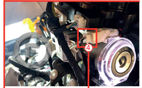
④ Close to key barrel. Près du barillet de clé.
