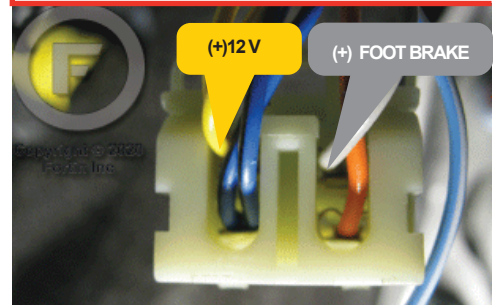
⑤ At brake switch Au commutateur de freins
