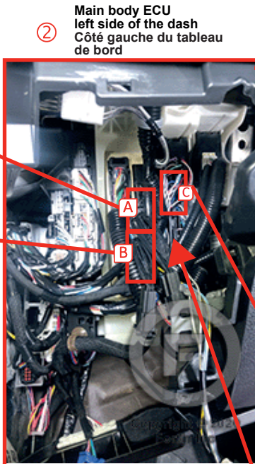
2C With stop and start system (Look for button in center console) Avec système stop et start (Regardez pour bouton à la console centrale)
