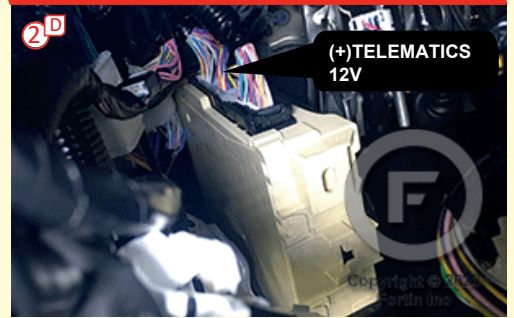
Without stop and start system Sans système stop et start At the back of the Main body ECU - below dash fuse box Au dos du Main body ECU - sous le tableau de bord
