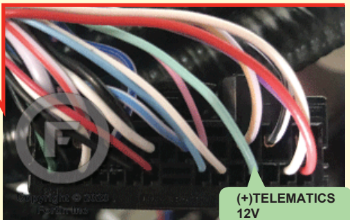
Without stop and start system Sans système stop et start At the back of the Main body ECU - below dash fuse box Au dos du Main body ECU - sous le tableau de bord
