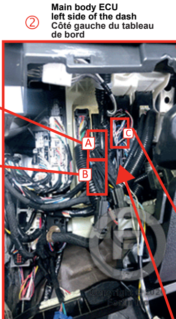
②C With stop and start system (Look for button in center console) Avec système stop et start (Regardez pour bouton à la console centrale)
