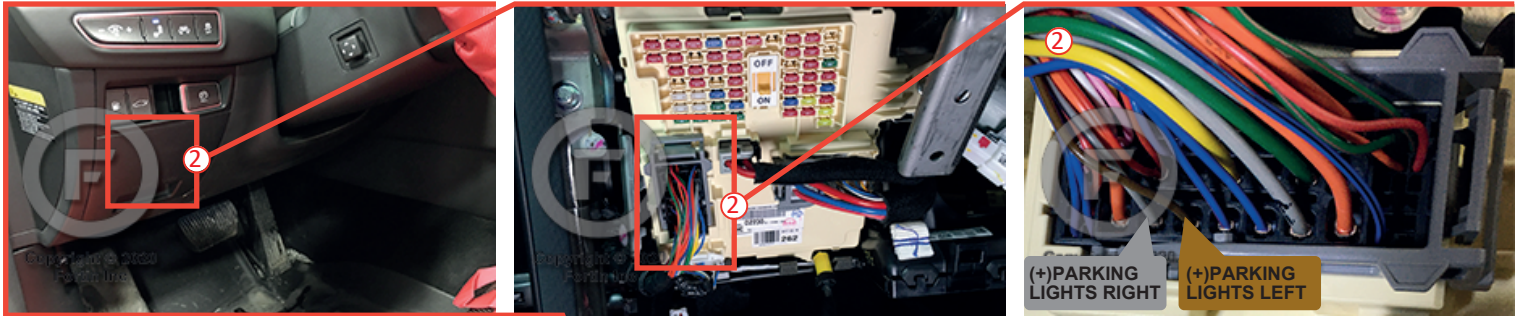
② Front of the fuse box Au devant de la boîte à fusibles
