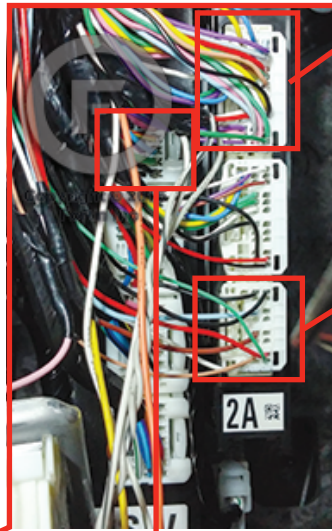
① BCM & smartKey module Behind fuse box BCM & Module de clé intelligente À l'arrière de la boîte à fusibles
