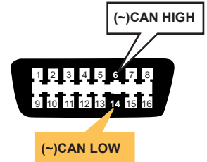
⑤ OBD-II connector. Connecteur OBD-II
