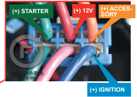
② Ignition harness Harnais d'ignition
