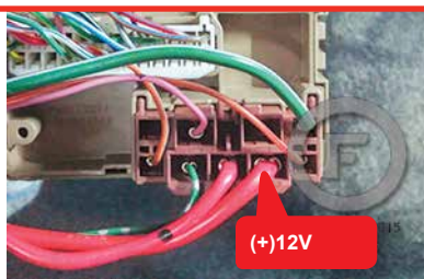
① Back of fuse box Au dos de la boîte à fusibles
