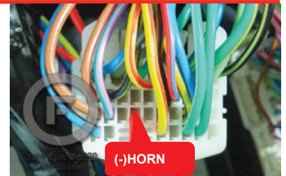
③C BCM Behind fuse box BCM À l'arrière de la boîte à fusibles
