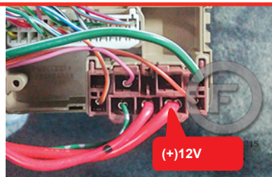
① Back of fuse box Au dos de la boîte à fusibles
