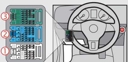
① Back view, 26-Pin White connector, at BCM. Vue de dos, connecteur Blanc 26-Pins, au BCM.
