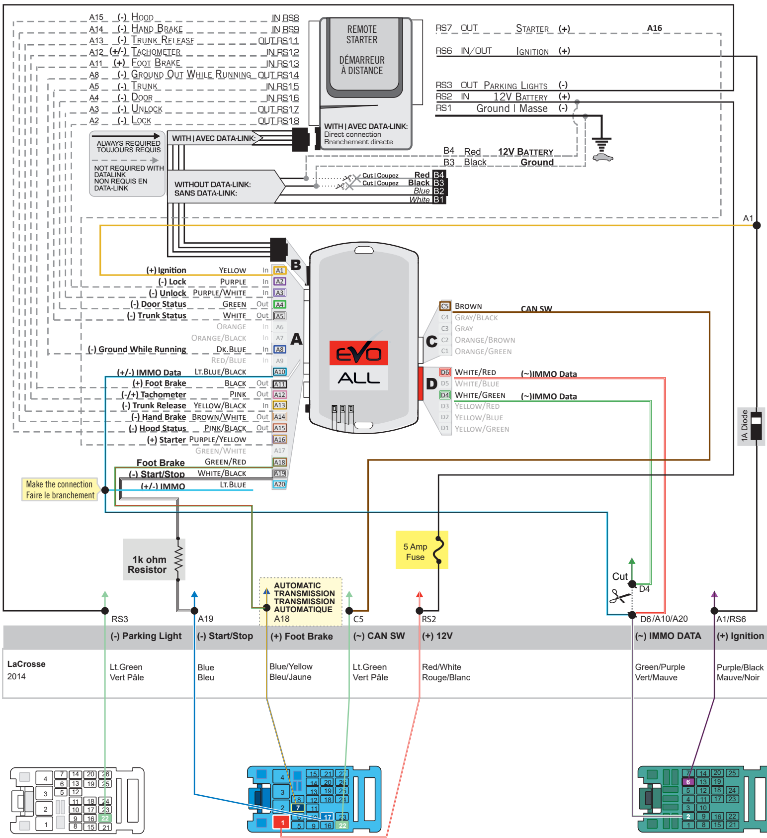
① Back view, 26-Pin White connector, at BCM. Vue de dos, connecteur Blanc 26-Pins, au BCM.
