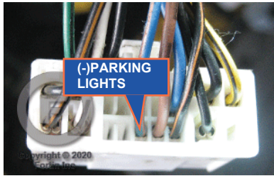
② At Parking light harness Au HArnais des feux de sttionnement
