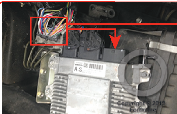
② ECM Engine compartment next to air cleaner assembly ECM Compartment moteur à côté du filtre à air
