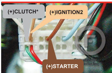
③B SmartKey module Behind fuse box Module de clé intelligente À l'arrière de la boîte à fusibles
