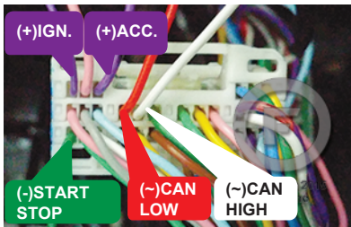
③A SmartKey module Behind fuse box Module de clé intelligente À l'arrière de la boîte à fusibles
