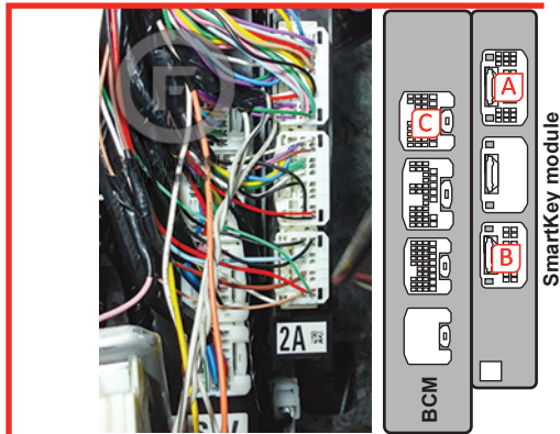
③ BCM & smartKey module Behind fuse box BCM & Module de clé intelligente À l'arrière de la boîte à fusibles
