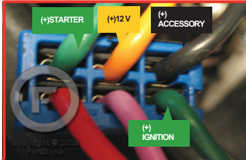
① At Ignition harness Au Hanais d'ignition
